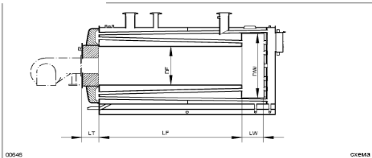
Размеры топки котла GKS-Dynatherm с тремя газоходами
